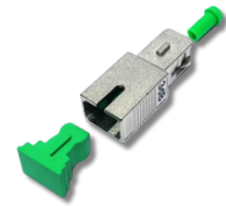
Atenuador APC SC Macho x SC Fêmea NX-SJQSCAXX Clip e trava do tipo ESC Conector óptico reutilizável
