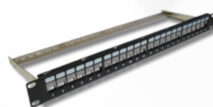
NX-2224A Painel Blindado Descarregado para Rack 19, 1U, 24 portas
